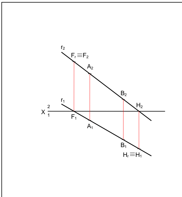
Representação de uma recta r e dos seus traços horizontal e frontal
