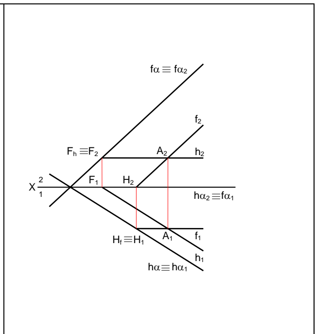
Representação de um plano α pelos seus traços horizontal e frontal e duas rectas horizontal e frontal do plano
