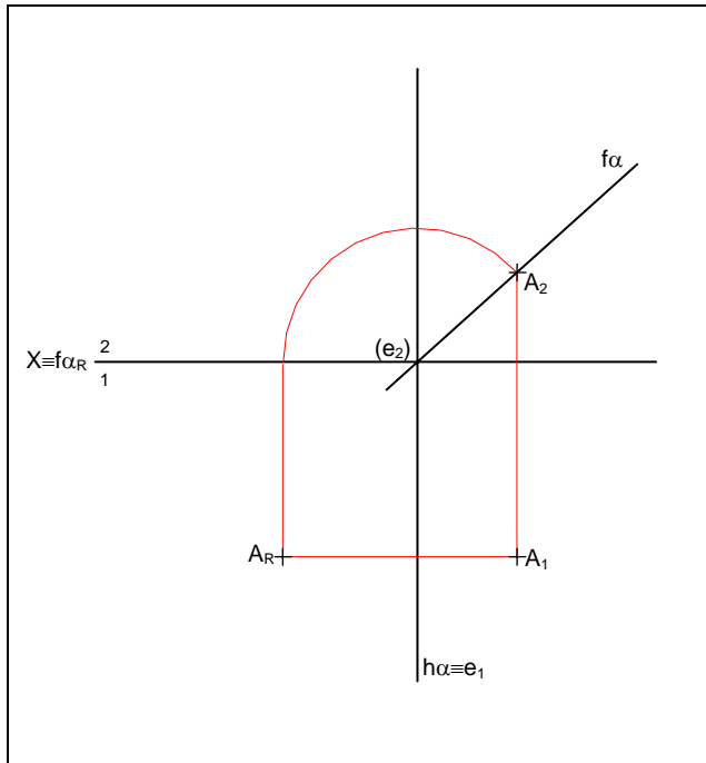
Rebatimento de um plano de topo em torno do seu traço horizontal
